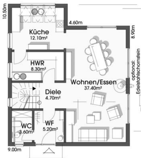
Erdgeschoss 1:175 71.30 m 2
