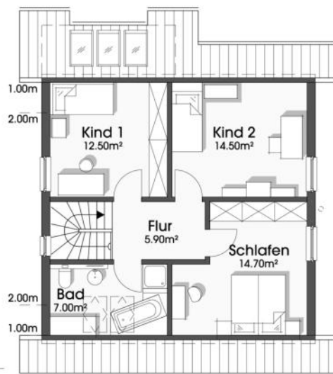
Dachgeschoss 1:175 54.40 m 2
